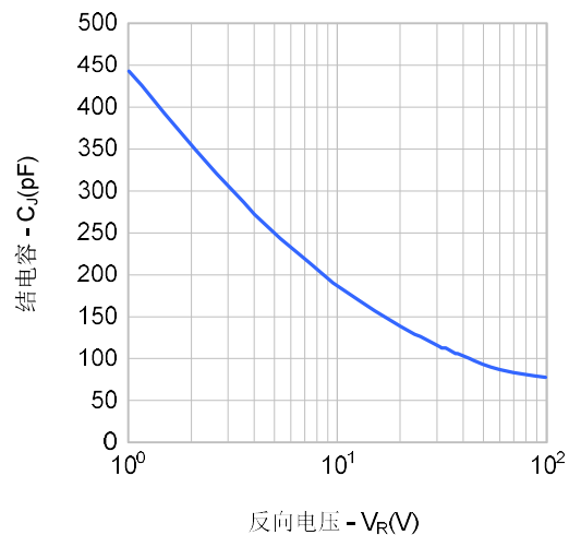
图 4. 结电容特性
